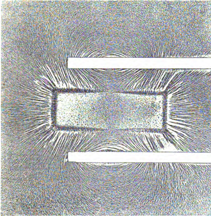
Abb. 108. Induktion eines prismatischen Eisenstückes im Felde eines Solenoides.
